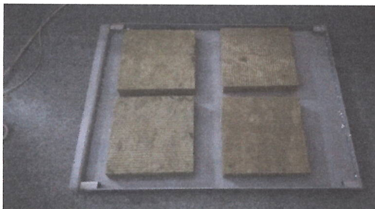
Рисунок 7 – Зволоження дослідних зразків теплоізоляційного матеріалу марки «РОКЛАЙТ ЛАЙТ»
